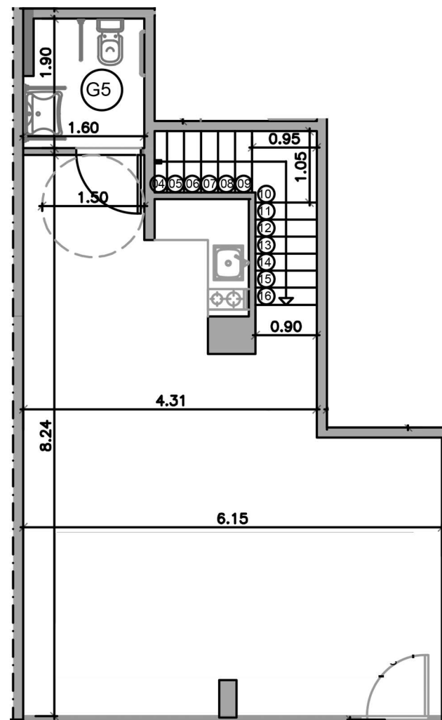
Planta Baja
